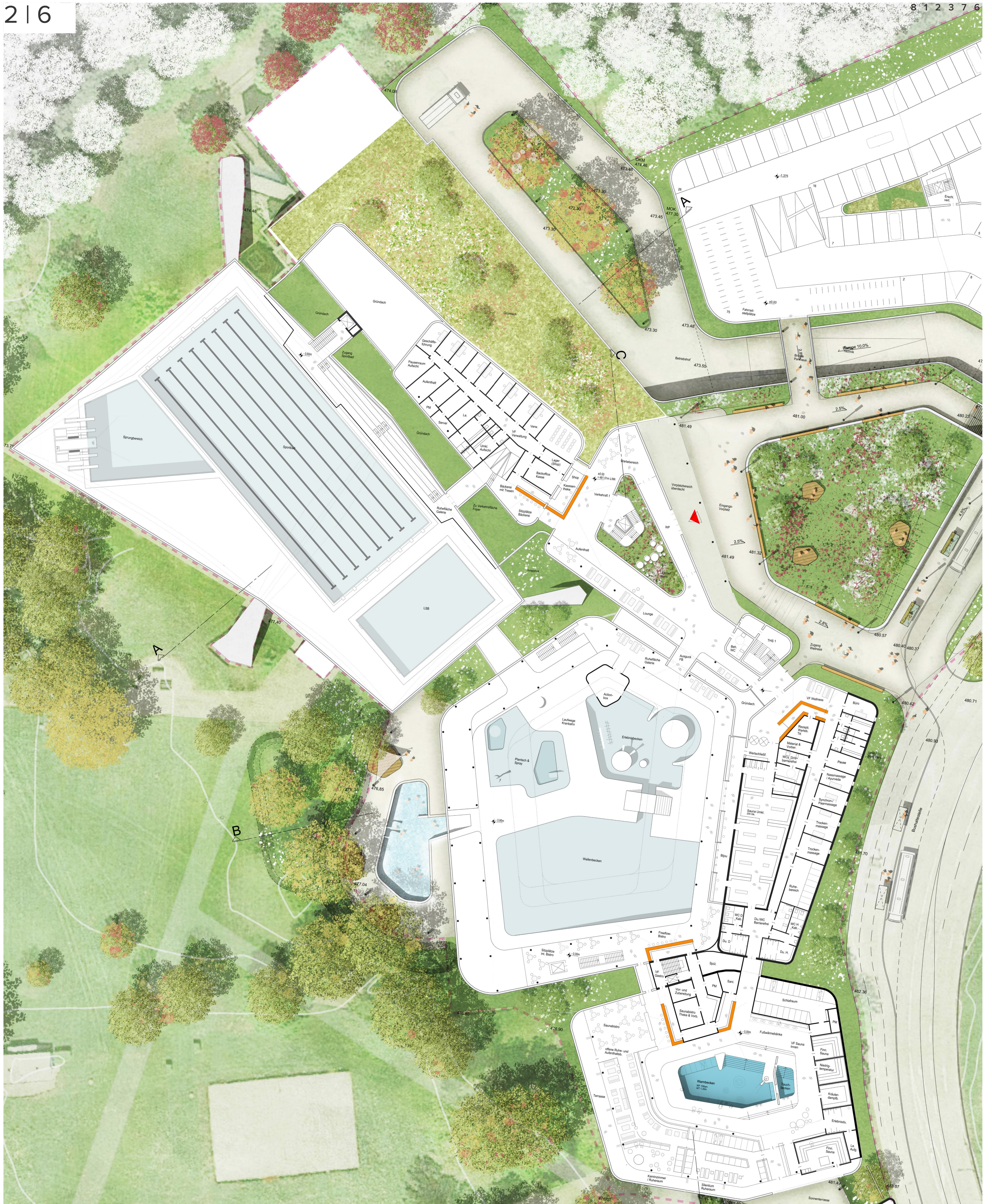
GRUNDRISS EINGANGSEBENE M 1:200
